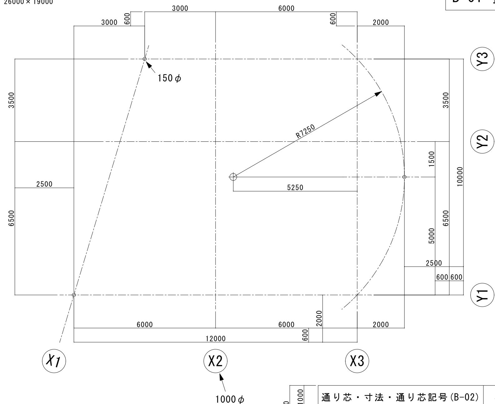
B-01 参考図
